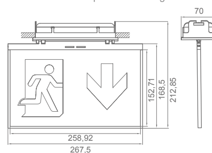
Inbouw plafondmontage
