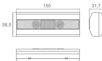
Opbouw Alya
