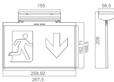
Opbouw plafondmontage
