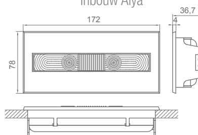
Inbouw Alya
