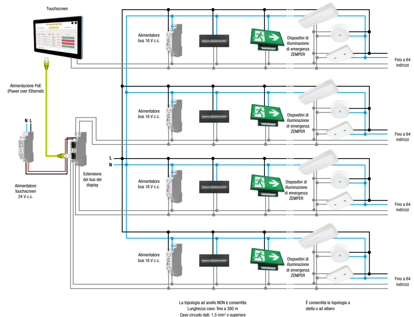
Figura 2. Bus multiplo (massimo 256 dispositivi di illuminazione)
