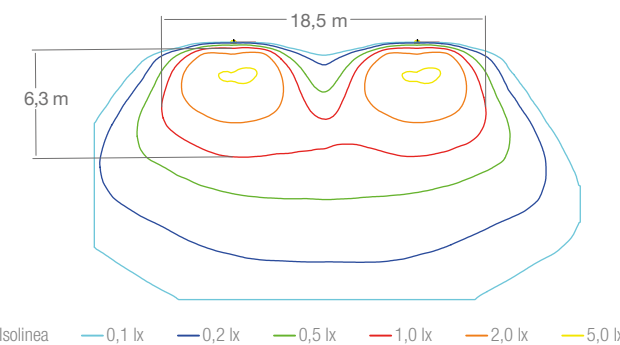
CURVA ISOLUX Dispositivo di illuminazione da 250 lm posizionato a 3 m di altezza
