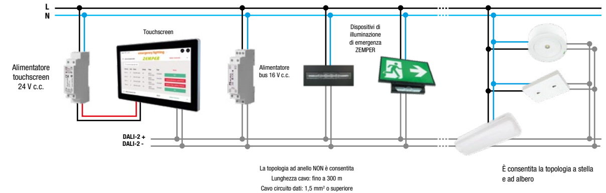
Figura 1. Bus singolo (massimo 64 dispositivi di illuminazione)
